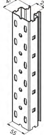
55B Upright
